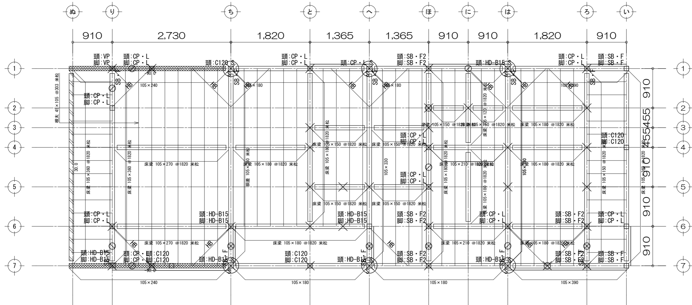
2階 床伏図 S:1/50
