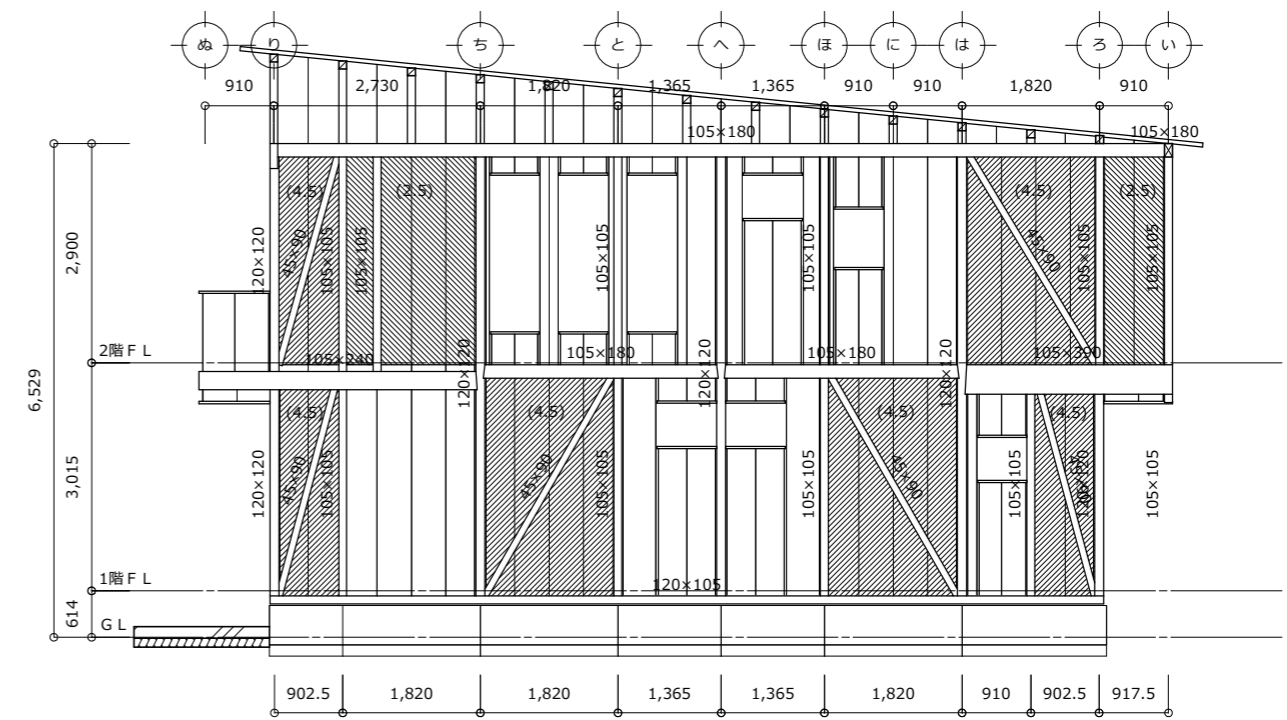
7通り軸組図
