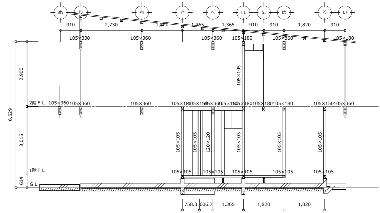
5通り軸組図
