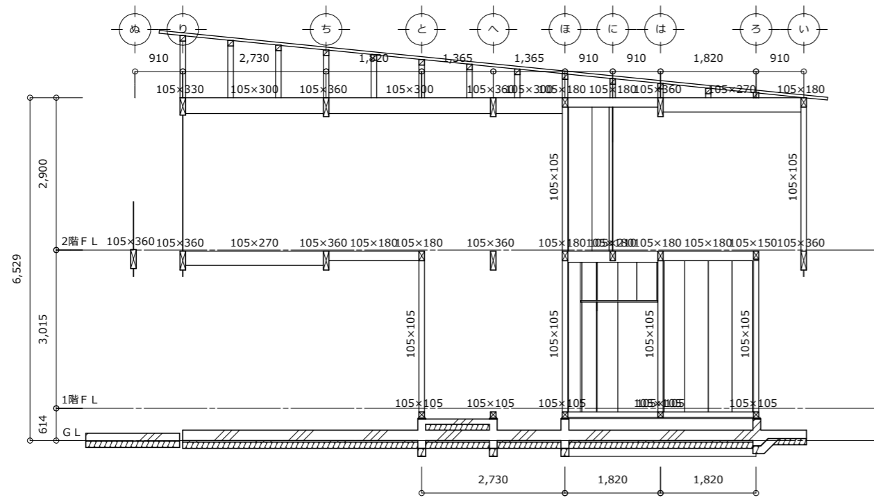
4通り軸組図
