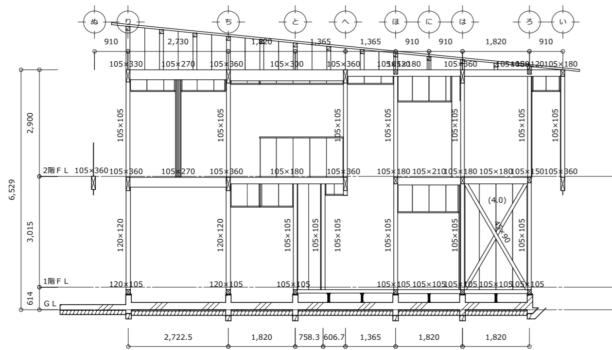
6通り軸組図
