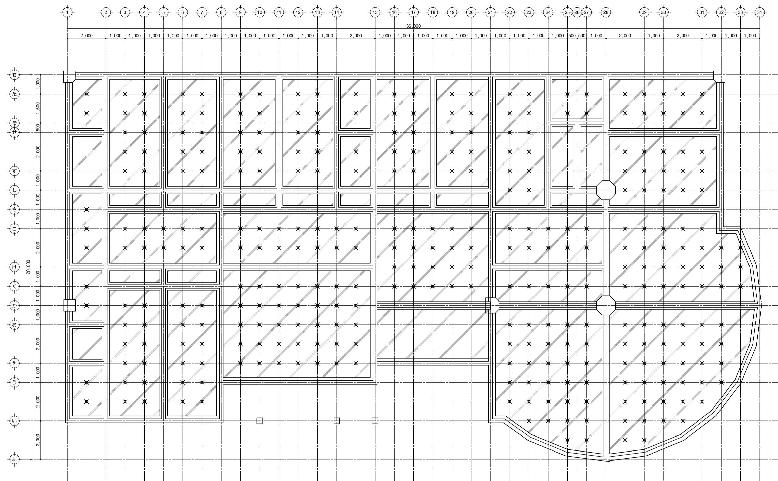
1F基礎伏図 1/100
