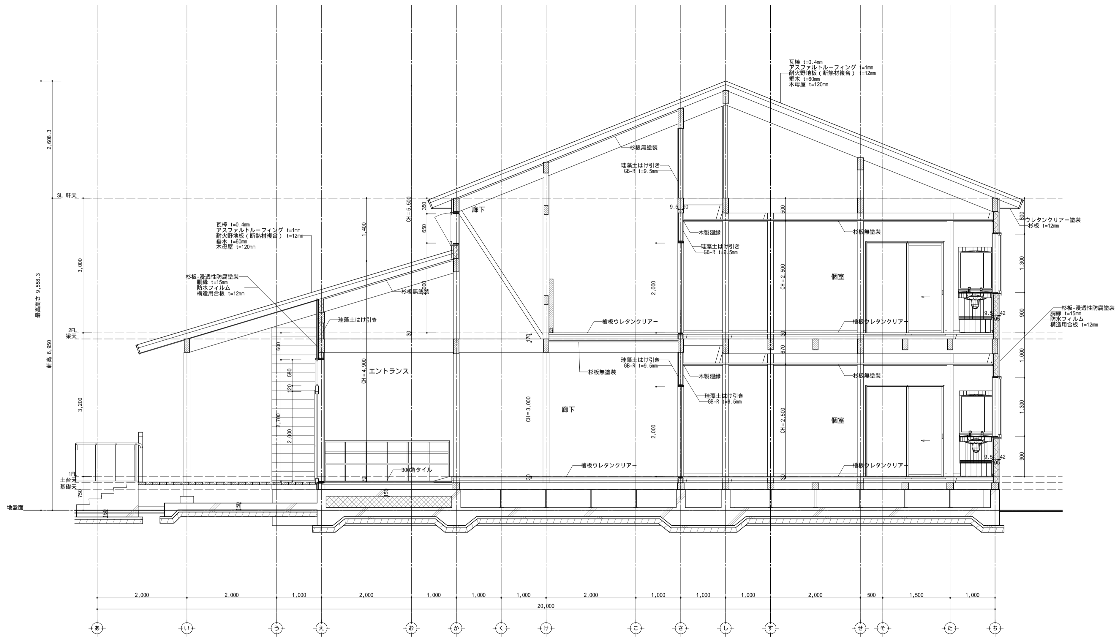
矩計図 1/50
