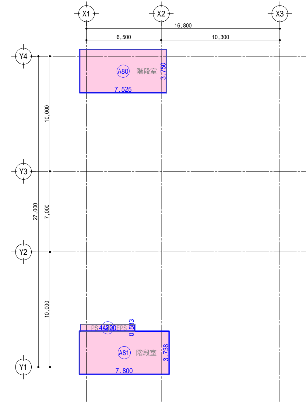
PH1床面積求積図 1/200
